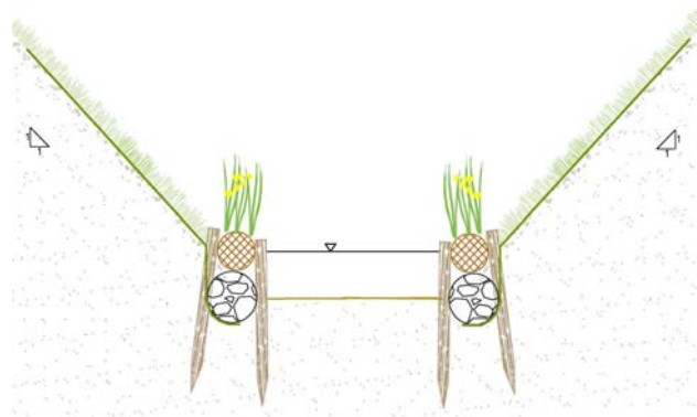
Imatges de la riera a l'inici dels treballs, i l'esquema de l'actuació amb la geomalla permanent, el gabió flexible fixant la geomalla i estabilitzant la base, i el Fiber Roll™ vegetatitzat.
